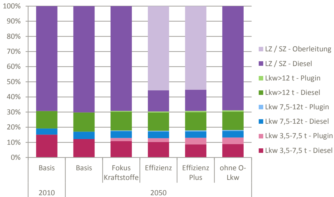
Abbildung 6-6: Lkw-Fahrleistung differenziert nach Antriebstyp und Größenklasse im Jahr 2050
