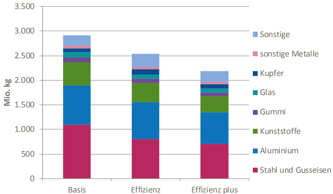
Abbildung 10-20: Materialeinsatz in der Pkw-Herstellung im Jahr 2050
